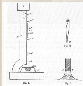
Schemat metody Czochralskiego pochodzi z artykułu z Zeitschrift für Physikalische Chemie 92, 219-221 (1918)
